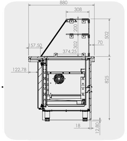
Ölçü Detayları Dimension Details
