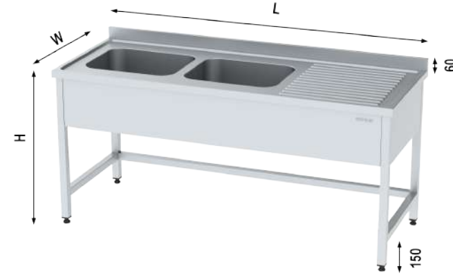
ÇİFT EVYELİ ÇALIŞMA TEZGAHI ALT TABLASIZ WORK TABLE WITH DOUBLE SINK WITHOUT BOTTOM
