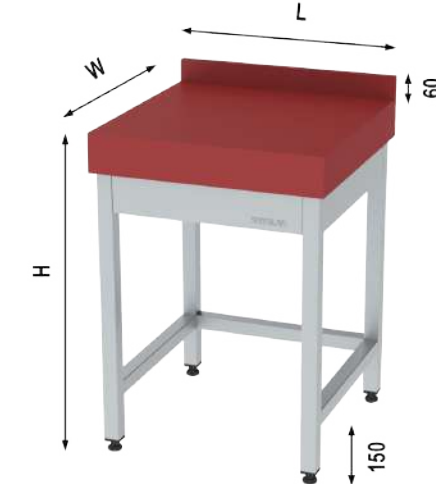
POLİETİLEN TABLALI ET KÜTÜĞÜ POLYETHYLENE TOP MEAT CHOPPING TABLE
