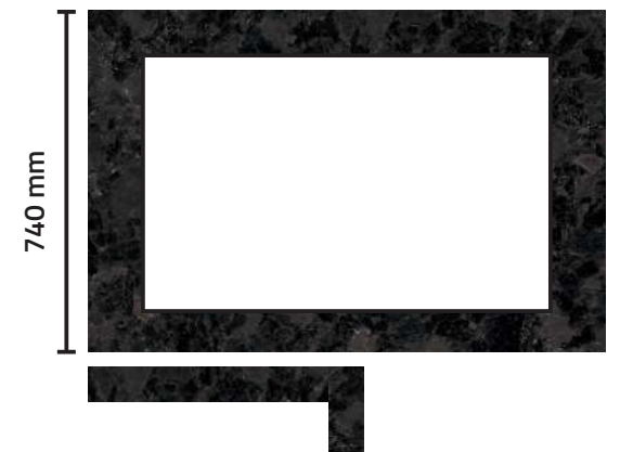
SELF SERVİS GRANİT TABLA (Hazneli Ürünler İçin)
