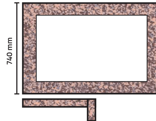
SELF SERVİS GRANİT TABLA (Hazneli Ürünler İçin)
