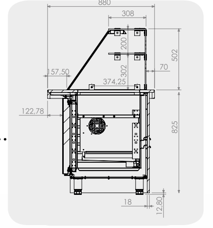
Ölçü Detayları Dimension Details
